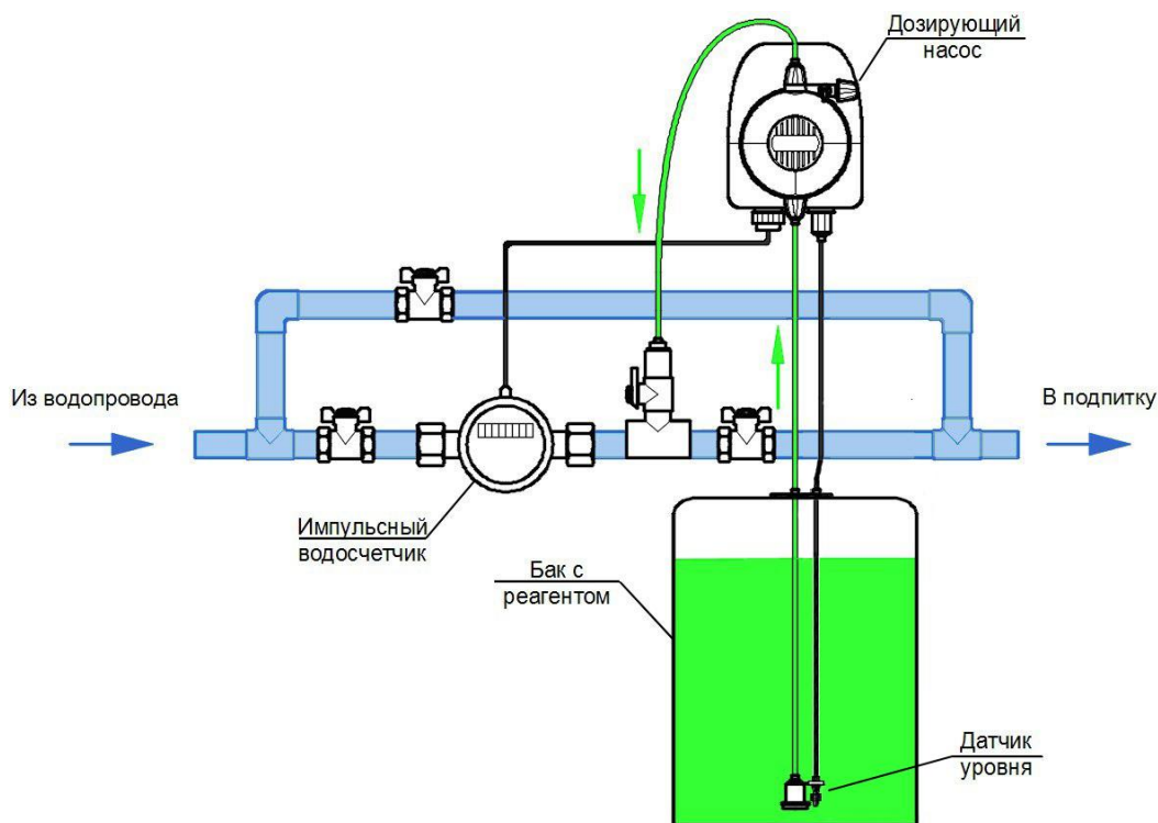
Схема монтажа станции дозирования на объекте
